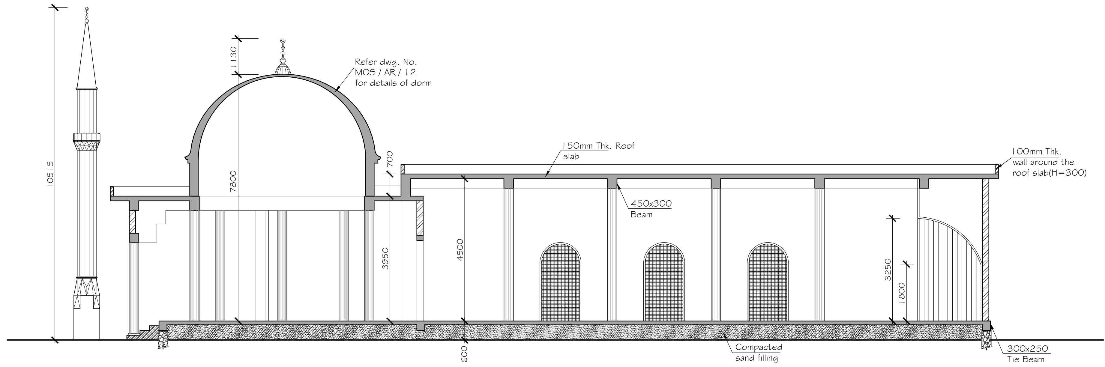
SECTION A-A
